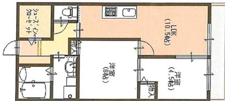
【間取り図】
