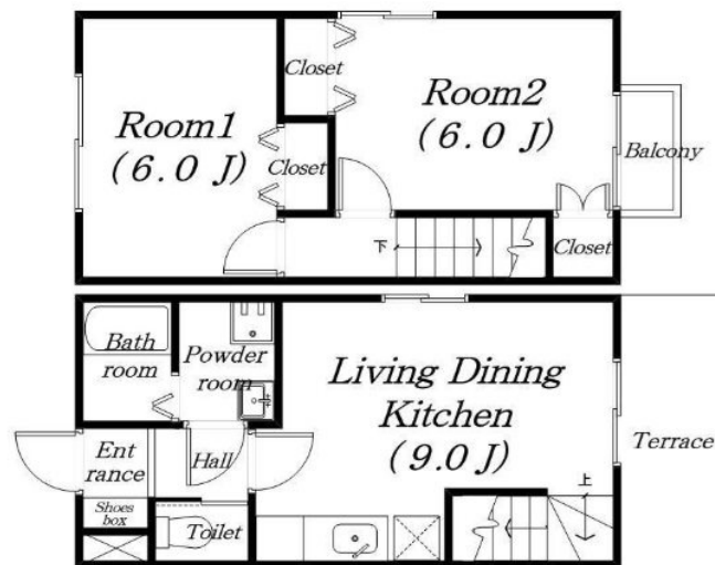
【間取り図】
